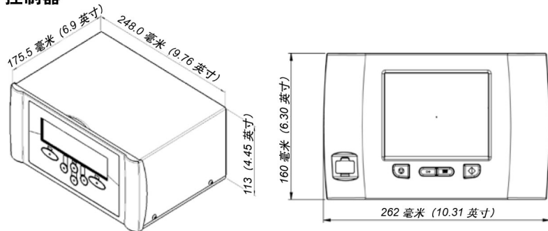
控制器
