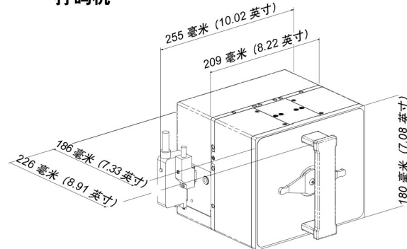
打码机
